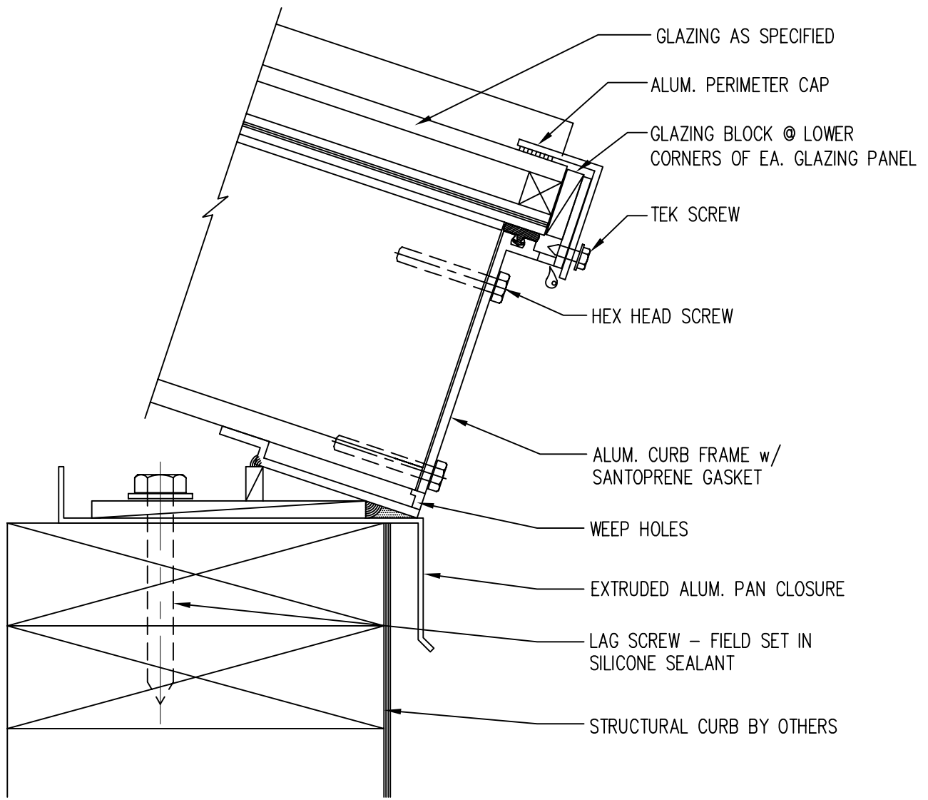
SILL SECTION F1 HALF SCALE
